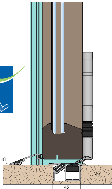
Coupe partie basse (seuil à encastrer)
