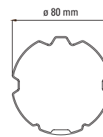
Adaptateur pour tube zf 80
