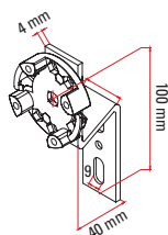
Support avec dépassement 40 mm
