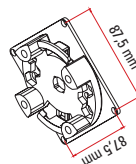
Support pour côtés Thyssen max 20 Nm
