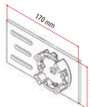
Support monobloc côté moteur
