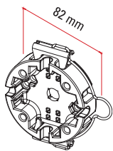
Support aluminium avec ressort de retenue
