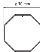
Adaptateur pour tube octogonal 70
