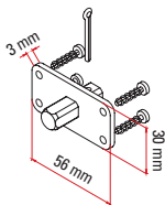
Support Axe carré 10 mm
