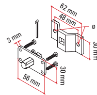
Kit support patte et axe carré 10 mm (trous passants)
