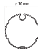
Adaptateur pour tube ogive 70
