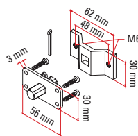
Kit support patte et axe carré 10 mm (trous taraudés)
