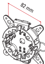
Support aluminium avec ailes et ressort de retenue
