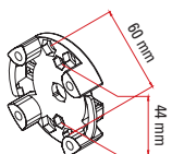
Support pour pattes ZF entraxe 44 max 20 Nm
