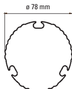
Adaptateur pour tube ogive 78 ou 3 ogives 78
