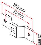
Support patte pour axe carré 10 mm
