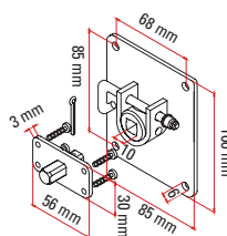
Kit support plaque 85 x 100 avec déverrouillage et axe carré 10 mm
